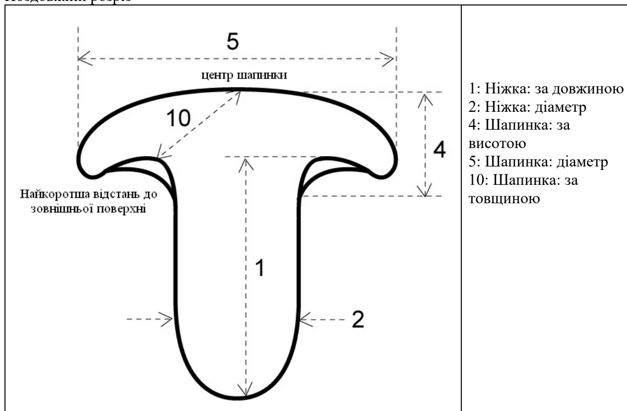
Приклад 3 Поздовжній розріз
