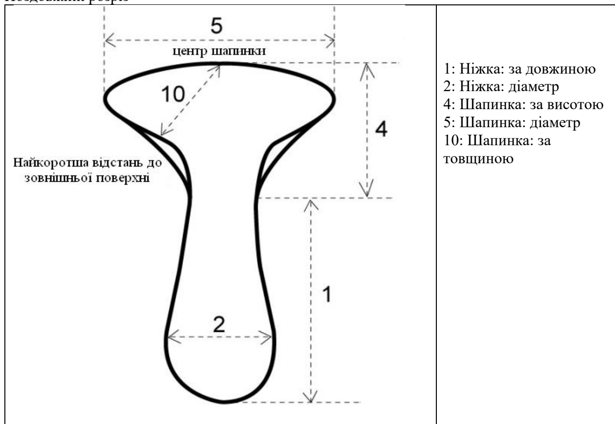
Приклад 3 Поздовжній розріз
